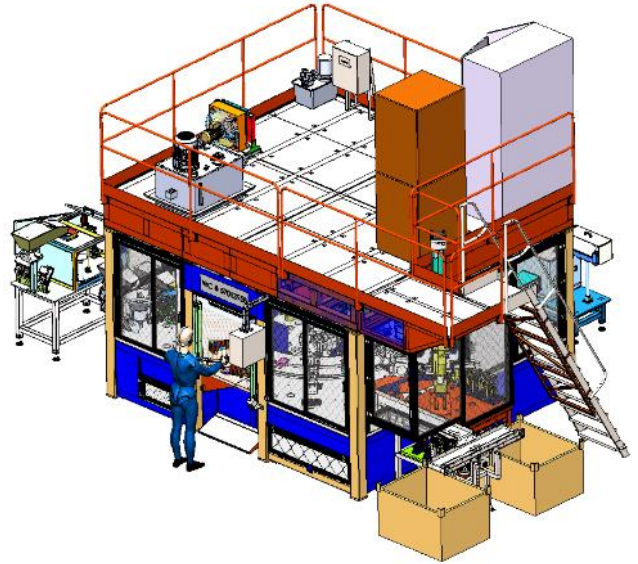
Dibujo de un diseño de una máquina rotativa de ensamble realizada por Jobitec DISEÑOS INDUSTRIALES.
